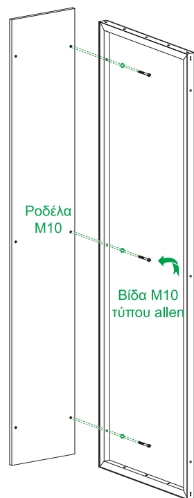
Σύνδεση πλαισίου με ορθοστάτη
