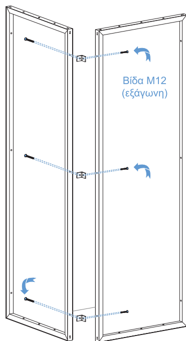
Σύνδεση πλαισίων υπό γωνία 90°
