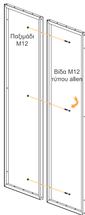
Σύνδεση πλαισίων σε ευθεία
